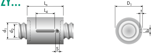
Zylindrische Mutter
