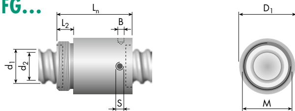
Flanschgewindemutter
